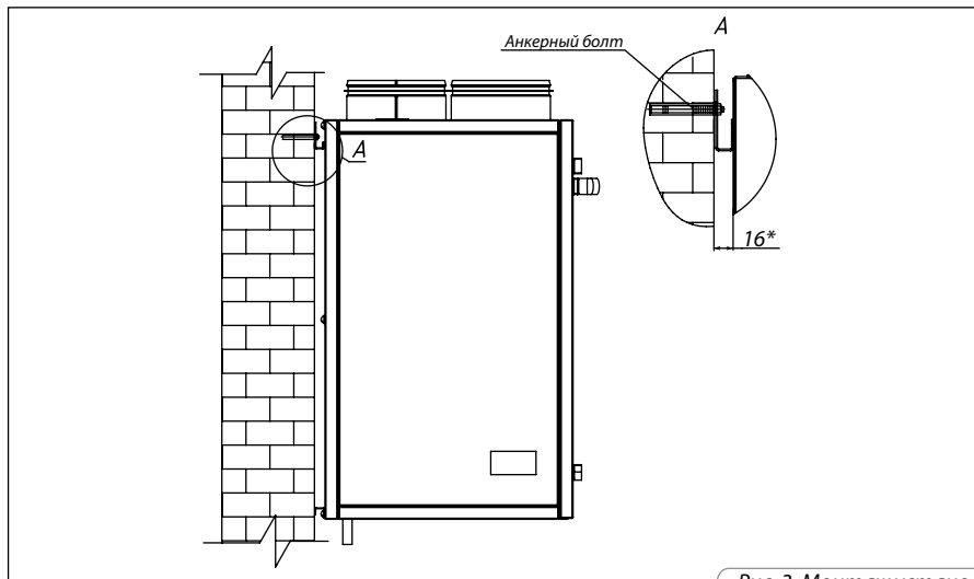
Рис. 3. Монтаж установки
