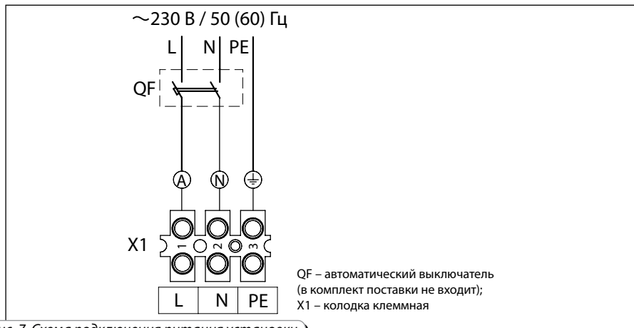
Рис. 7. Схема подключения питания установки
