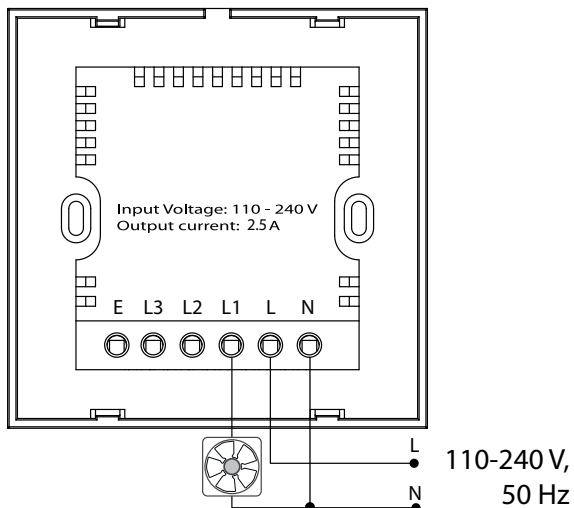
Wiring diagram (SGS E1 and SGS E2.5)
