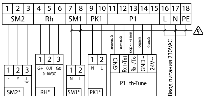
СХЕМА ВНЕШНИХ ПОДКЛЮЧЕНИЙ УСТАНОВОК KOMFORT ROTO EC L(E)HP S17
