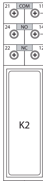
СХЕМА ПОДКЛЮЧЕНИЯ ВНЕШНЕГО НАГРЕВАТЕЛЯ
