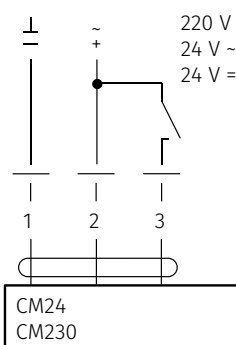
Однопроводное управление
