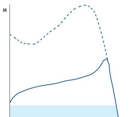
График крутящего момента при пуске от устройства плавного пуска
