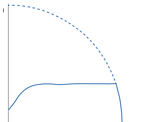
График тока при пуске от устройства плавного пуска
