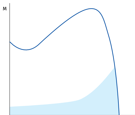
График крутящего момента при прямом пуске
