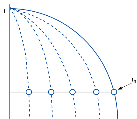
График тока при пуске от ПЧ
