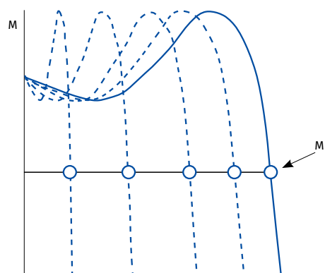
График крутящего момента при пуске от ПЧ
