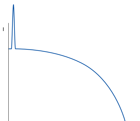
График тока при прямом пуске
