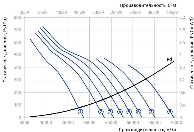
Типоразмер: 1000 Количество полюсов: 4
