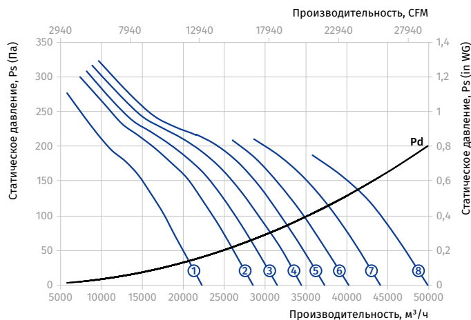
Типоразмер: 1000 Количество полюсов: 6
