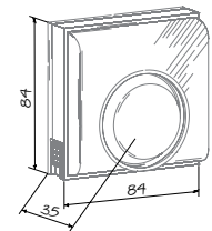
Термостат
