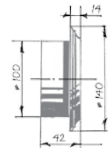
Круглая решетка
