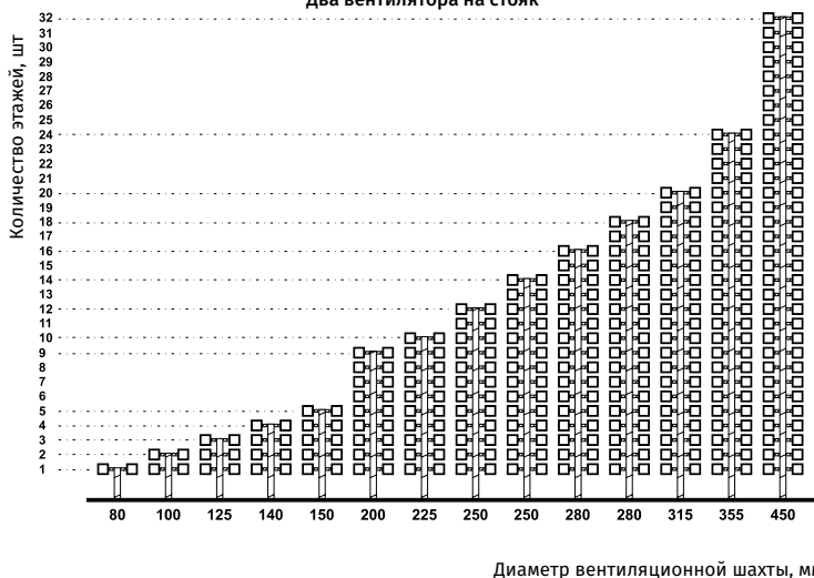
Два вентилятора на стояк
