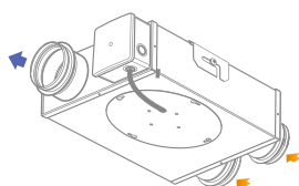
2 входных патрубка Ø 80 или 100 мм
