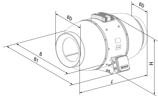
Iso-Mix EC 160 – Iso-Mix EC 315
