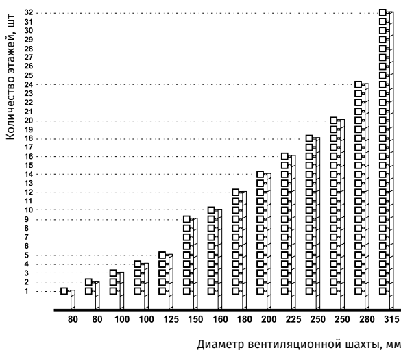
Один вентилятор на стояк
