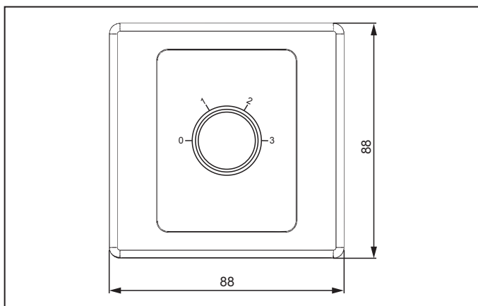
Рис. 1. Габаритные размеры
