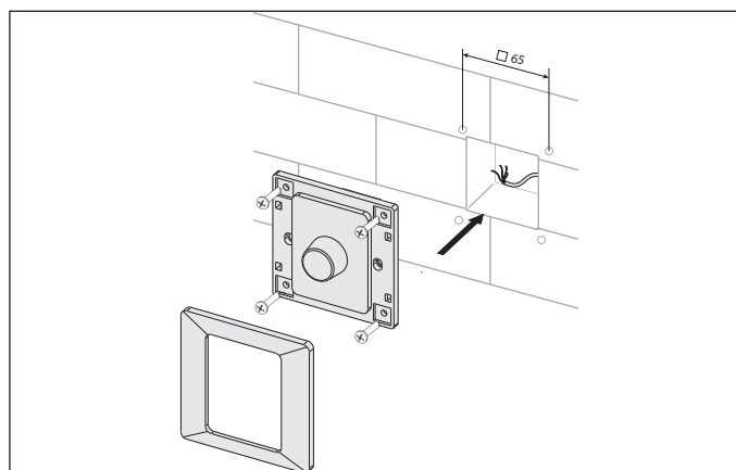
Рис. 2. Монтаж
