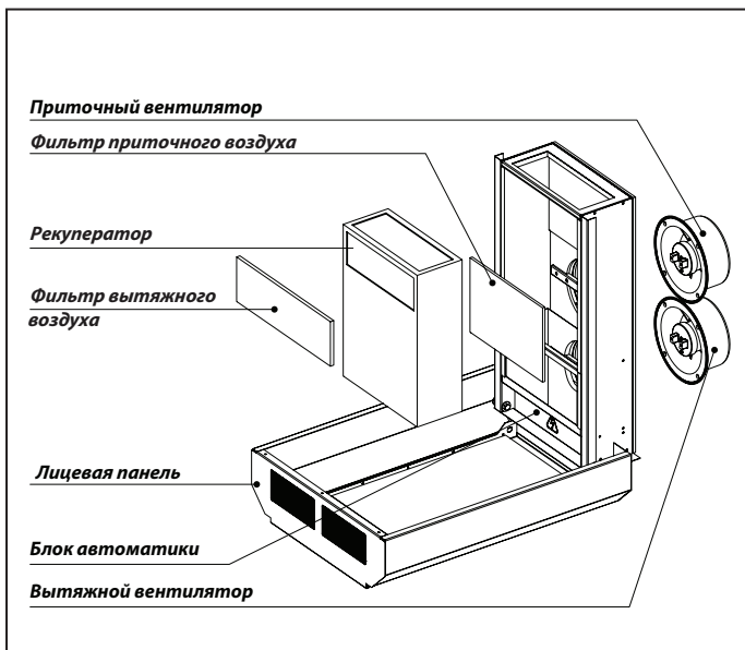
Рис. 1. Конструкция установки
