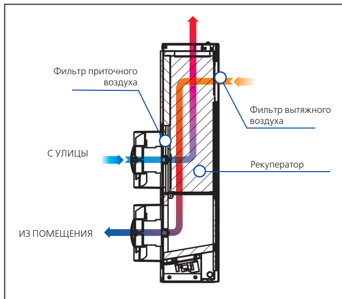
Рис. 2. Принцип работы
