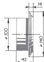
Круглая решетка
