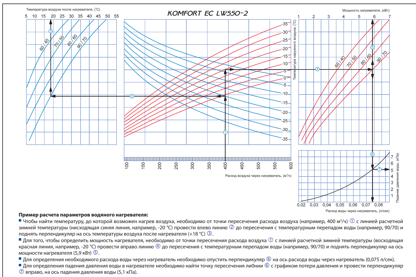
Рис. 4. Расчет водяного нагревателя KOMFORT EC LW550-2
