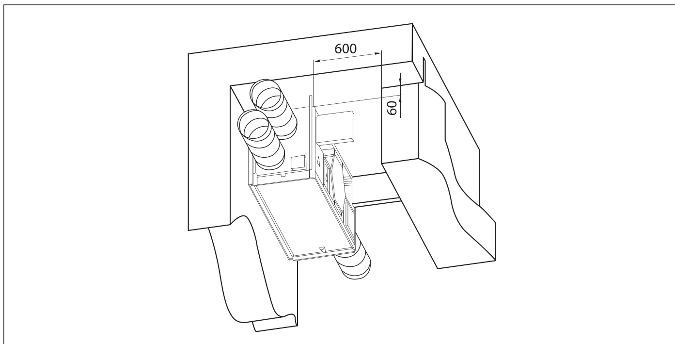
Рис. 5. Минимальное расстояние для техобслуживания
