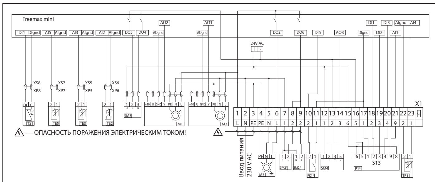
Рис. 10. Схема электрических подключений
