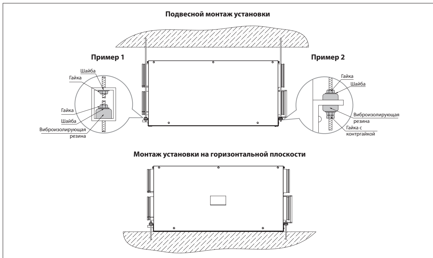
Рис. 6. Монтаж
