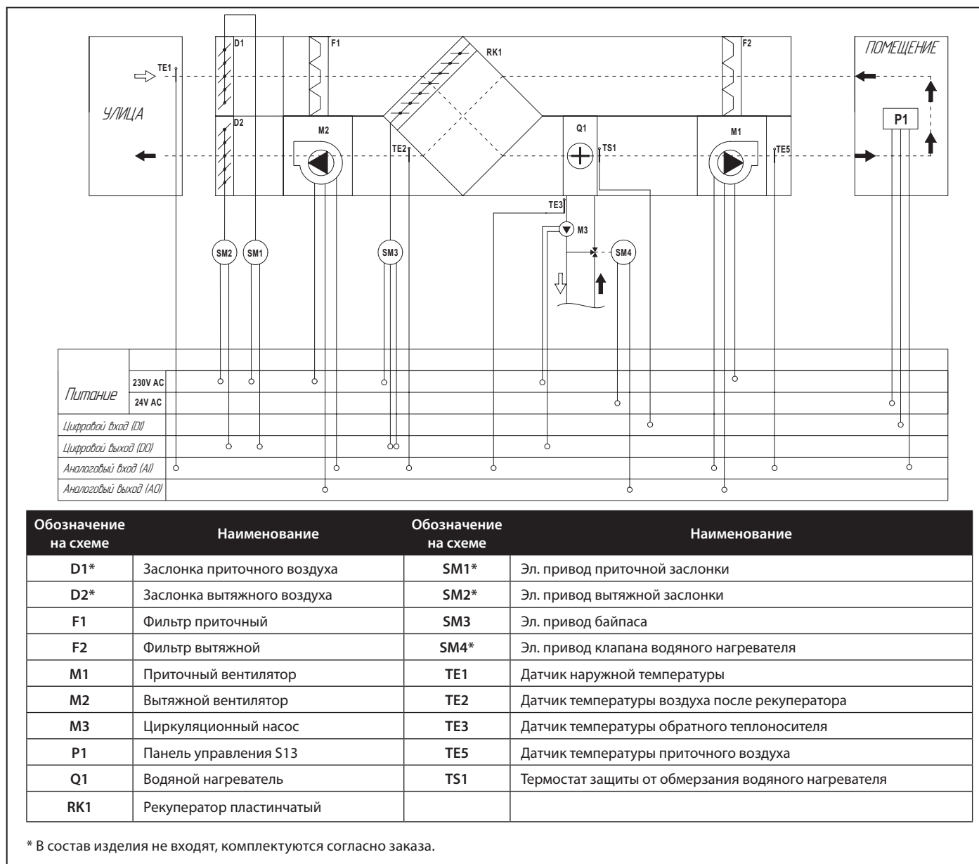
Рис. 11. Функциональная схема
