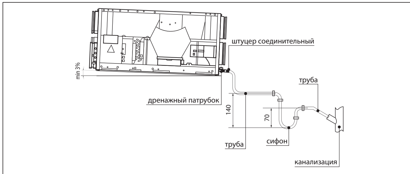
Рис. 9. Отвод конденсата
