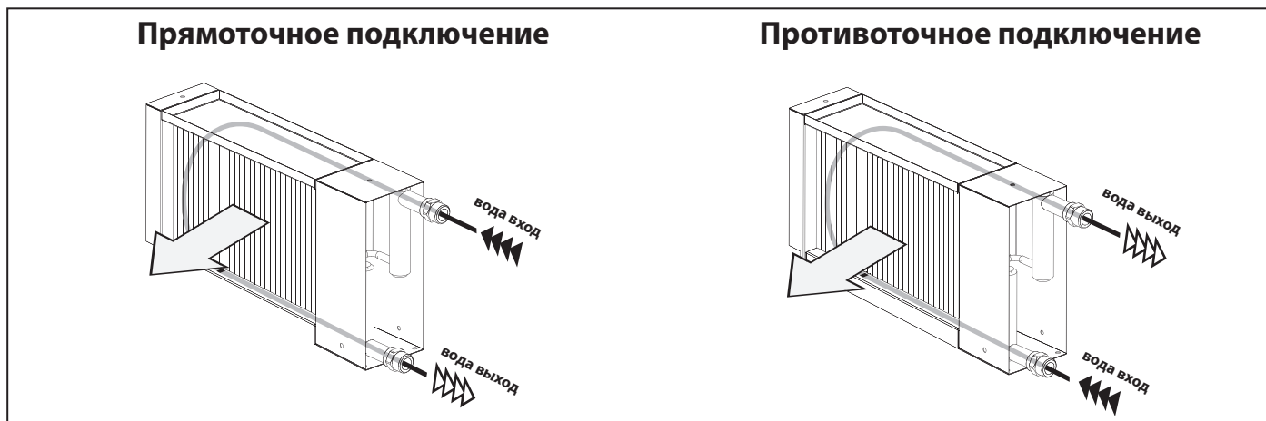
Рис. 7. Подключение водяного нагревателя
