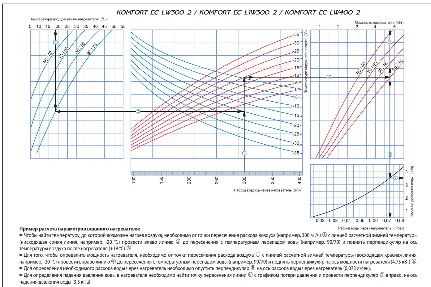
Рис. 3. Расчет водяного нагревателя KOMFORT EC LW300-2 / KOMFORT EC L1W300-2 / KOMFORT EC LW400-2
