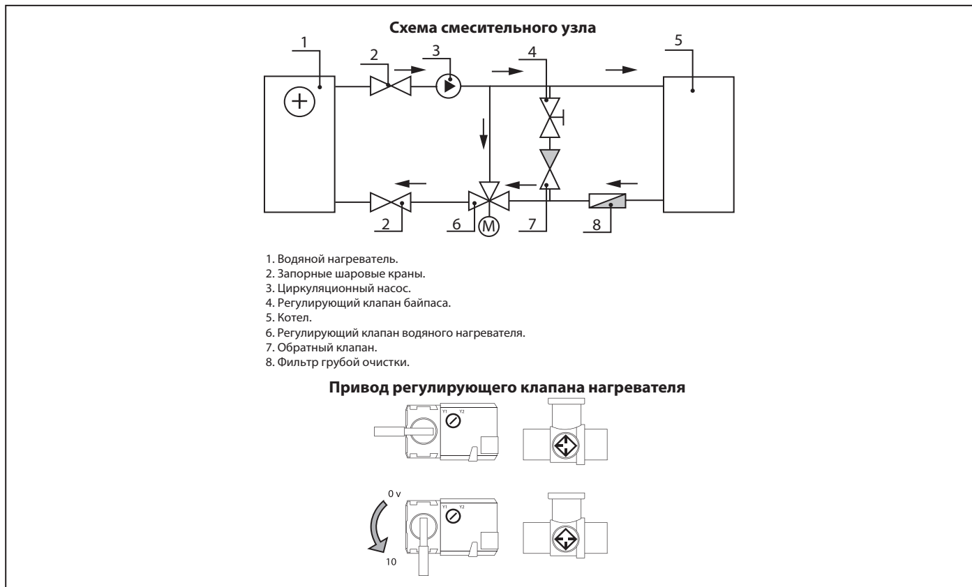
Рис. 8. Схема смесительного узла
