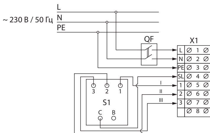
Рис. 4. Электрическая схема подключения
