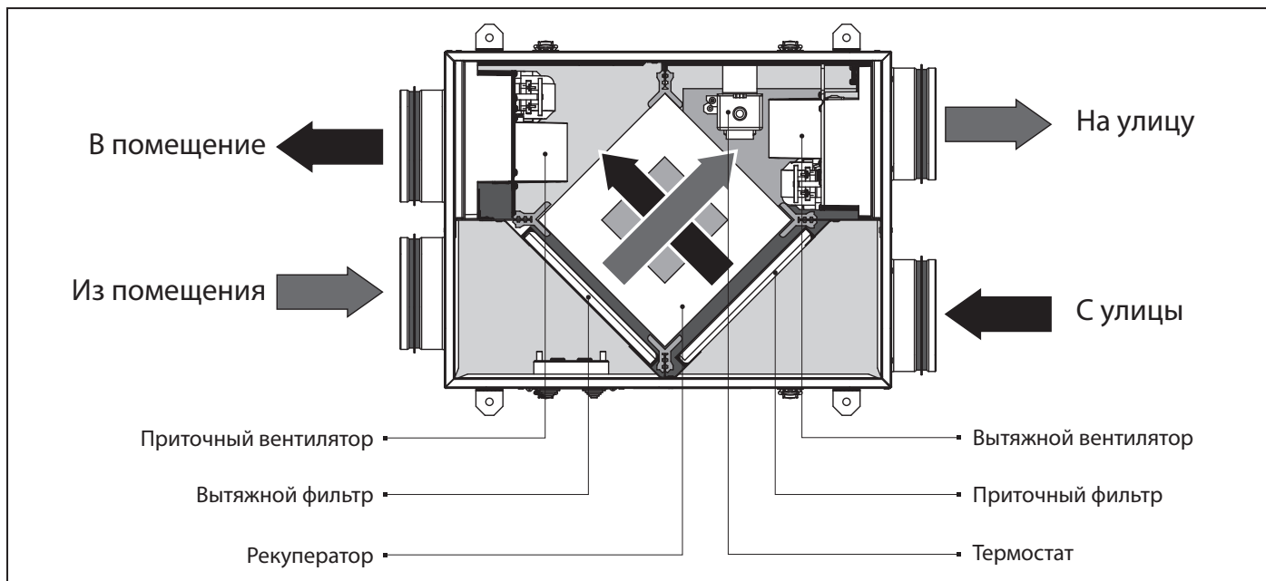
Рис. 1. Устройство и принцип действия установки
