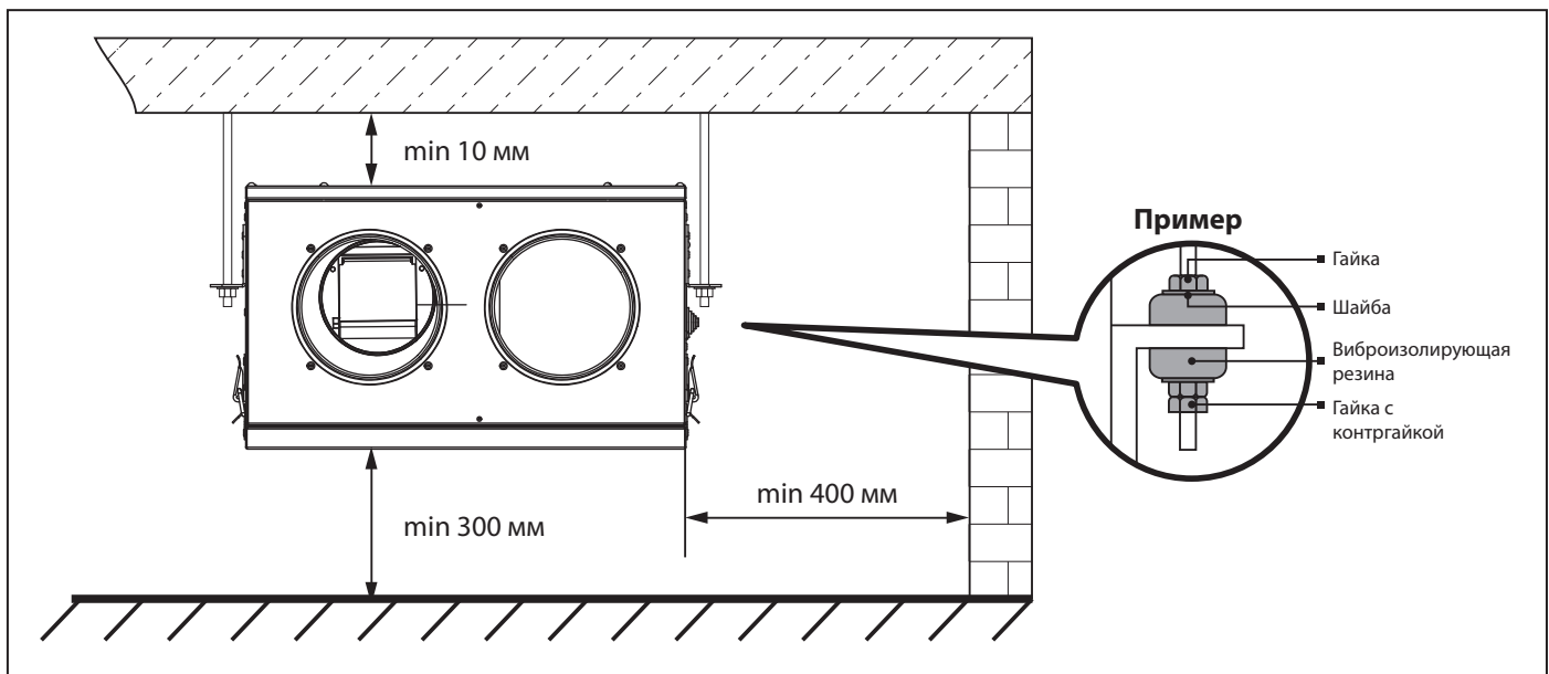
Рис. 3. Монтаж установки
